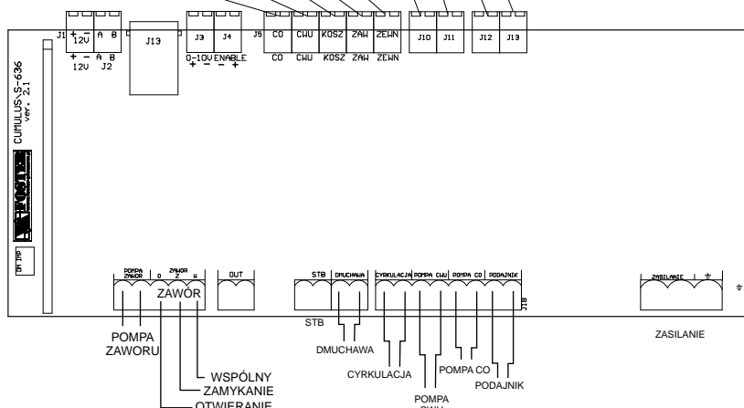
Rys.21. Widok płyty głównej z kostkami montażowymi do podłączenia urządzeń wejściowych i wyjściowych wersja 2019.
