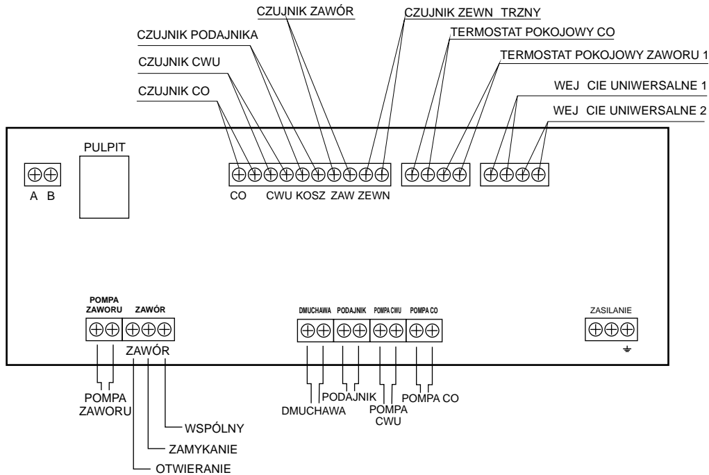
Rys.19. Widok płyty głównej z kostkami montażowymi do podłączenia urządzeń wejściowych i wyjściowych.
