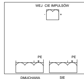
Rys.22. Widok płyty modułu HD z kostkami montażowymi (dotyczy sterowania CUMULUS HD)
