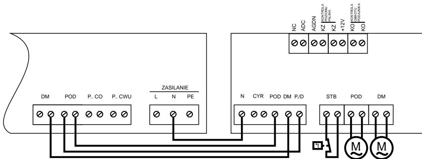
Rys.20. Widok płyty z kostkami montażowymi do podłączenia STB oraz urządzeń wejściowych i wyjściowych.
