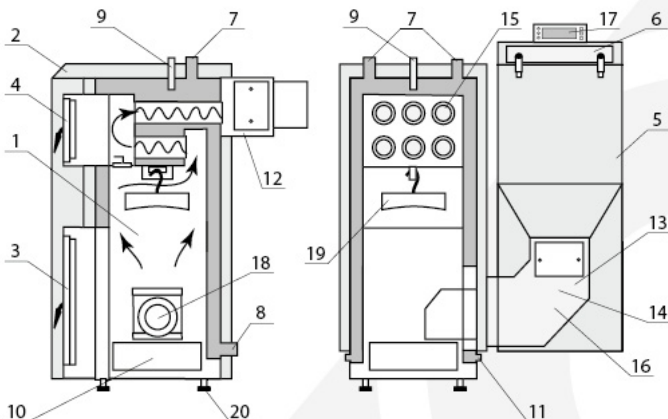
Kotły wodne typu KLAster-5P
