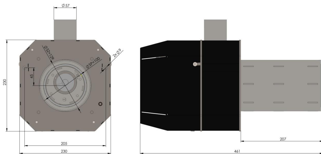
Rys. 23. Widok palnika 6-26 kW.
